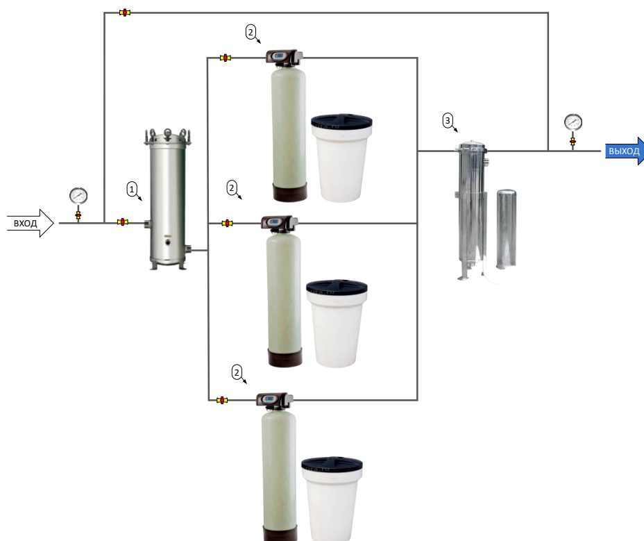
Рисунок 1 – Схема очистки воды методом умягчения
